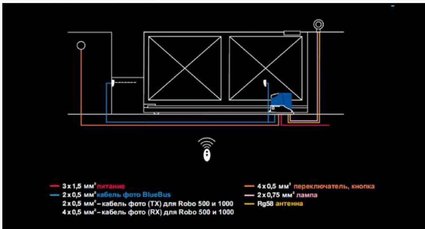
Схема проводки питания
